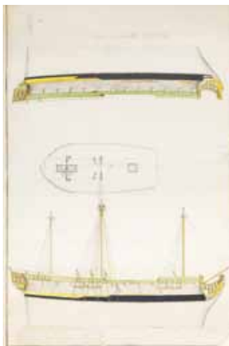
Илл. 7. Чертеж малой яхты, построенной для его императорского высочества в Гатчину, сочиненный корабельным подмастерьем Василием Сарычевым 27 июня 1792. Центральный военно-морской музей
