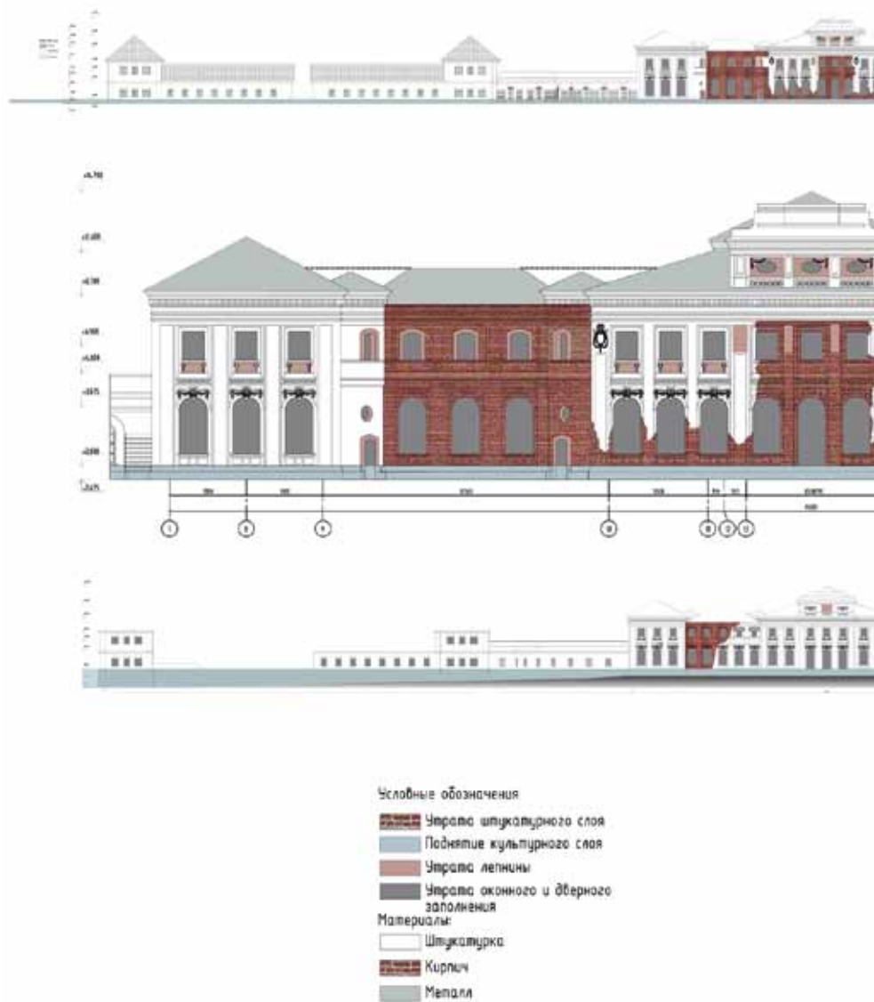
Илл. 2. Картограммы дефектов фасадов здания. Автор: Сходнова М.М.
